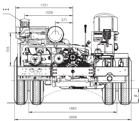
Tampak Belakang
